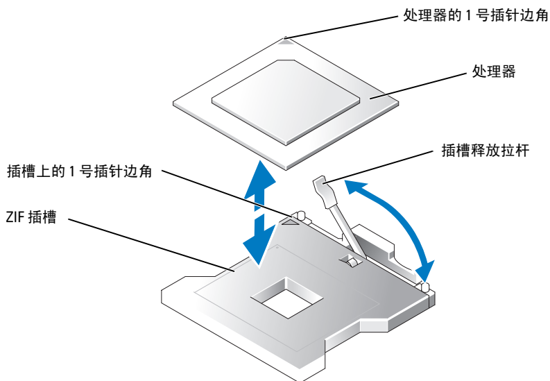
图 1-2. 装卸处理器
